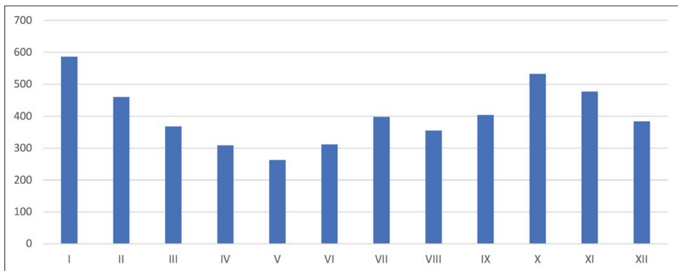
Ilość wykonanych badań próbek pasz w 2018 roku (Ogółem 4 849 próbek)
