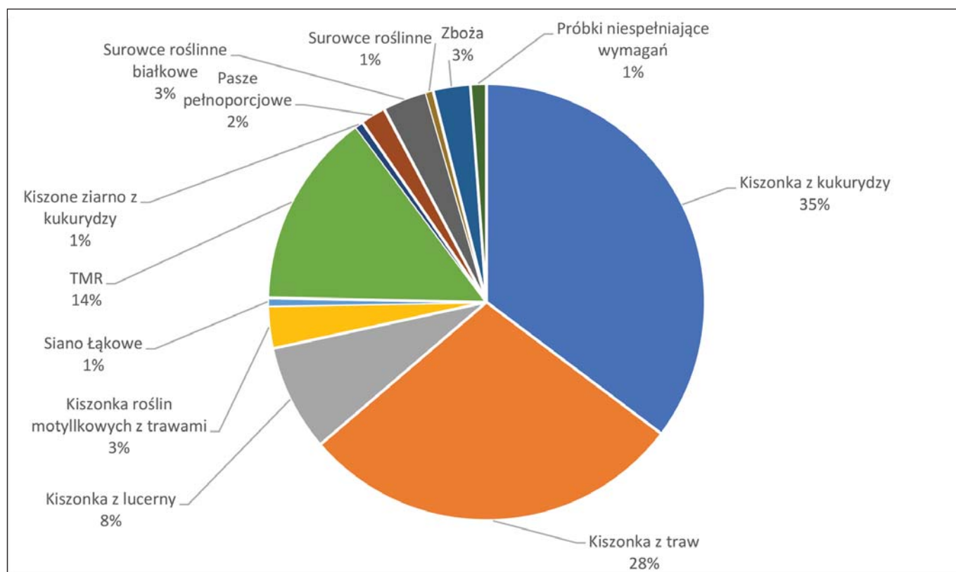
Procentowy udział próbek dla kalibracji pasz zbdanych w 2018 roku
