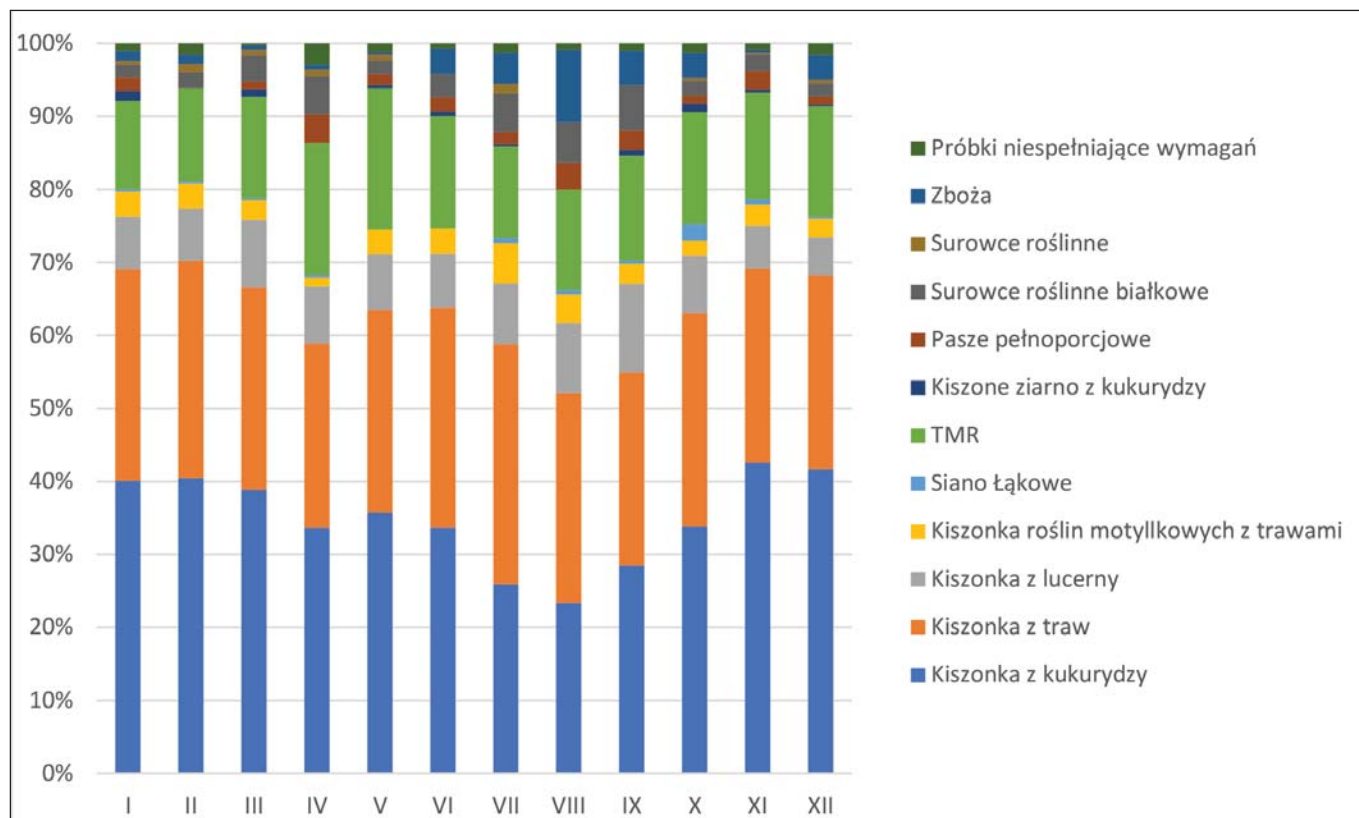
Procentowy udział próbek dla kalibracji pasz w kolejnych miesiącach 2018 roku
