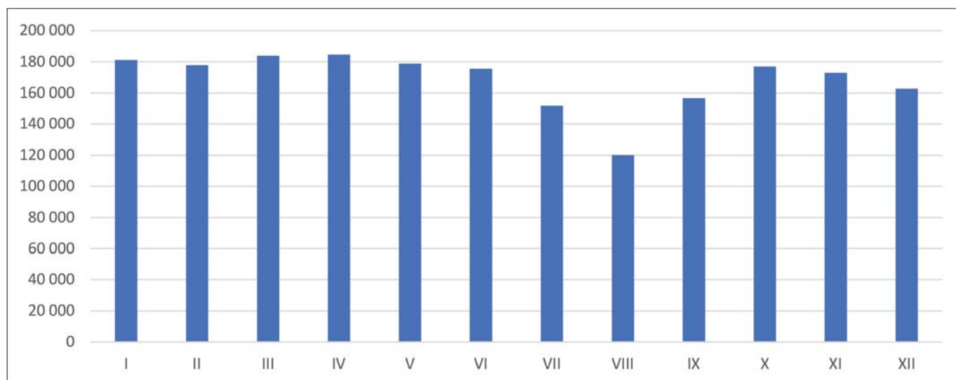
Ilość wykonanych badań próbek mleka w 2018 roku (Ogółem 2 023 297 próbek)
